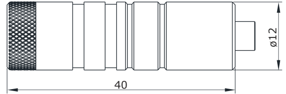
Hauptabmessungen Positioniereinsatz
