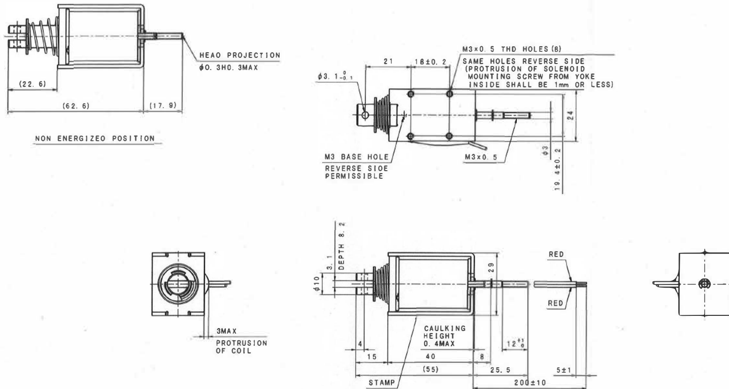
Masszeichnungen - Abmessungen in mm
