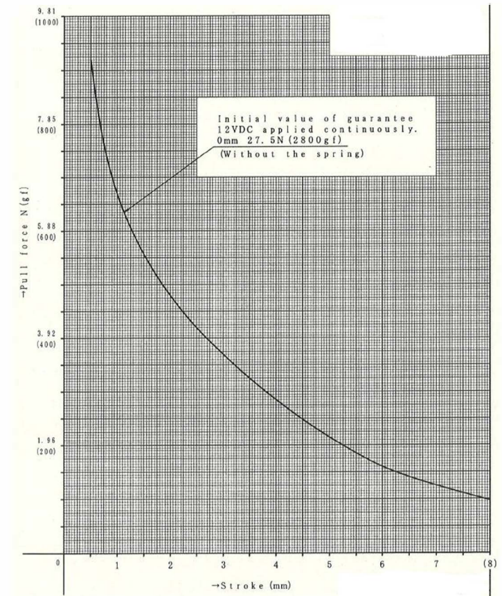
Kraft-Weg-Diagramm
